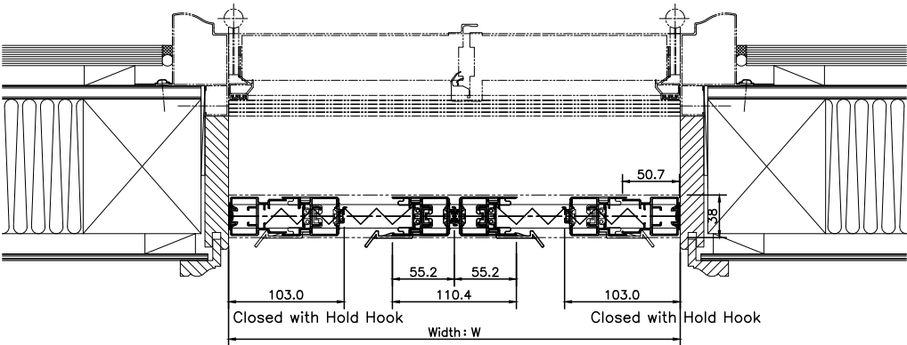
Caterpillar2 Double door (88L) Cross section
