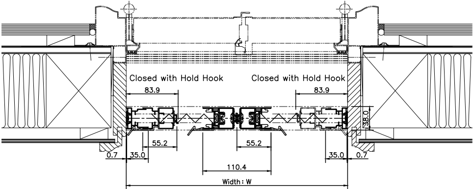
Caterpillar2 Double door (8LF) Cross section
