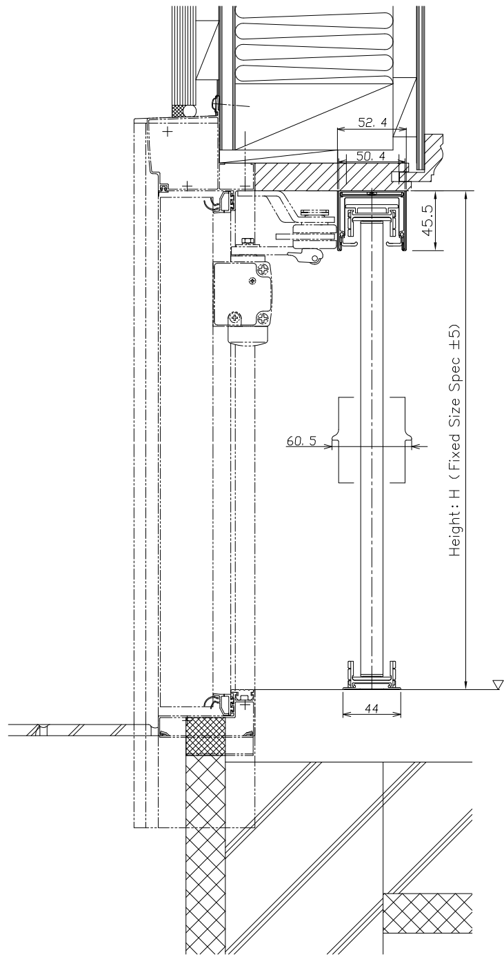
Senpooch Latch Type Longitudinal section
