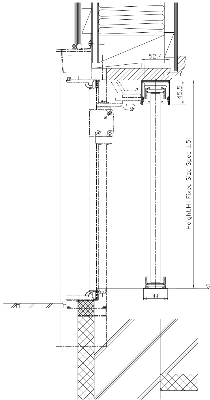
Senpooh Magnet Type Longitudinal section
