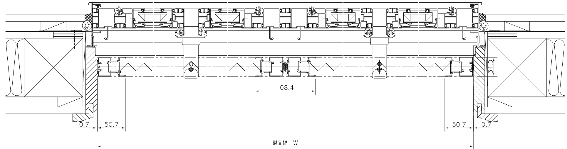
侍風 両引き (88LMEW) 横断面図
