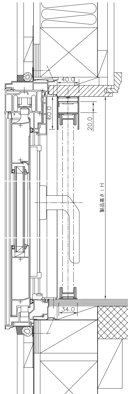
侍風 (88LMEW) 縦断面図
